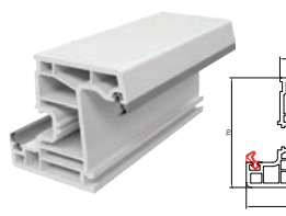
DÜZ KANAT PROFİLİ
